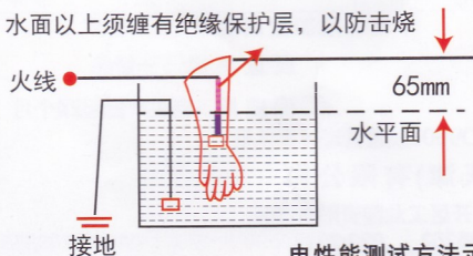
电性能测试方法示意图
